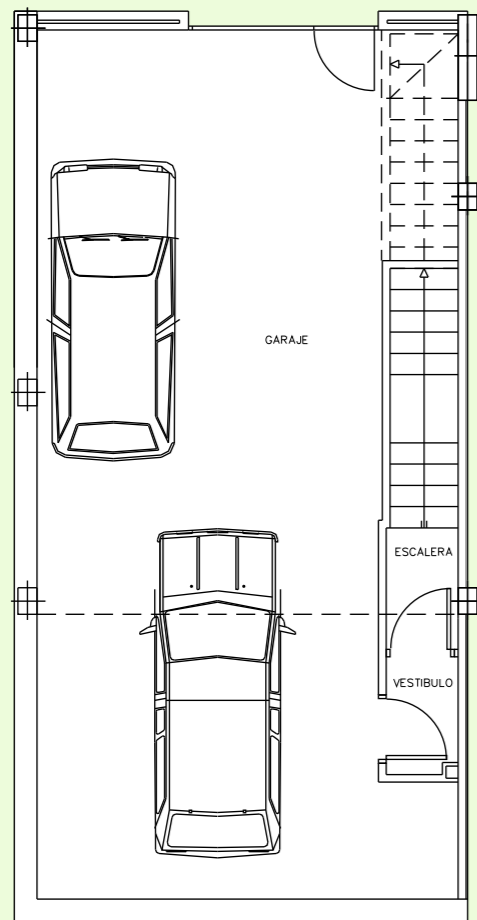
PLANTA SOTANO
